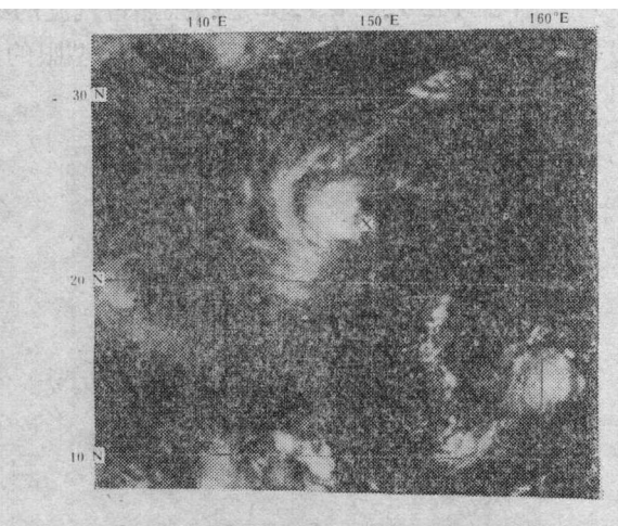
图 1 b 1978 年 9 月 12 日 14 时地球静止卫星红外云图。图上给出 7816 号台风发展初期的云系，环流中心位于强对流云区东侧边沿“×”所示的位置
