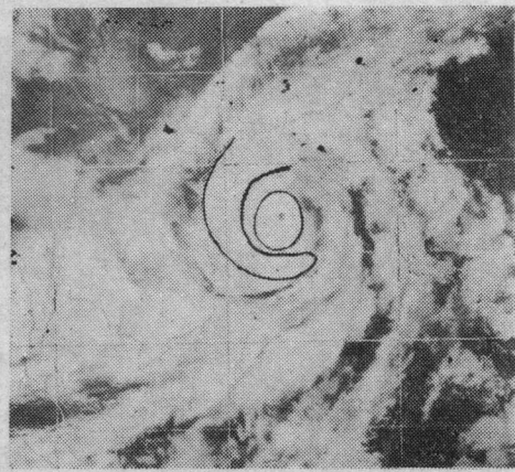
图 3f 1978年9月30日02时地球静止卫星红外云图。图上给出7818号台风的螺旋云系。围绕眼区是圆形中心强对流云带,它外面是外螺旋云带。
